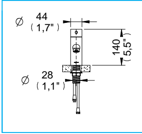
Medidas Referenciales / Estimated Dimensions, Acot.mm.(pulg) / Dim.mm.(in)
